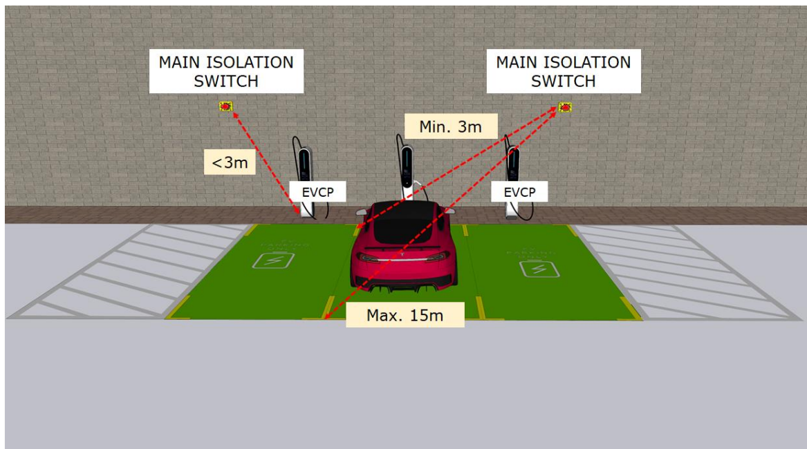
Rajah 12: Keperluan Tambahan Suis Pengasingan Elektrik Utama
