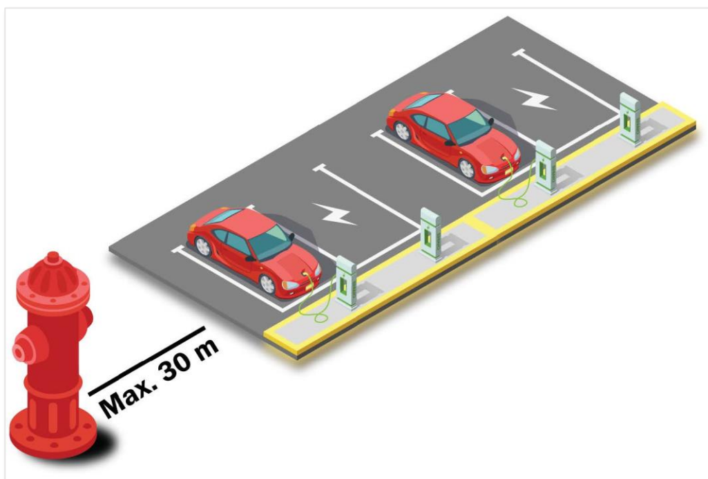
Rajah 9: Kedudukan EVCB Jenis Peranti DC Dari Wet Riser , Dry Riser atau Pili Bomba
