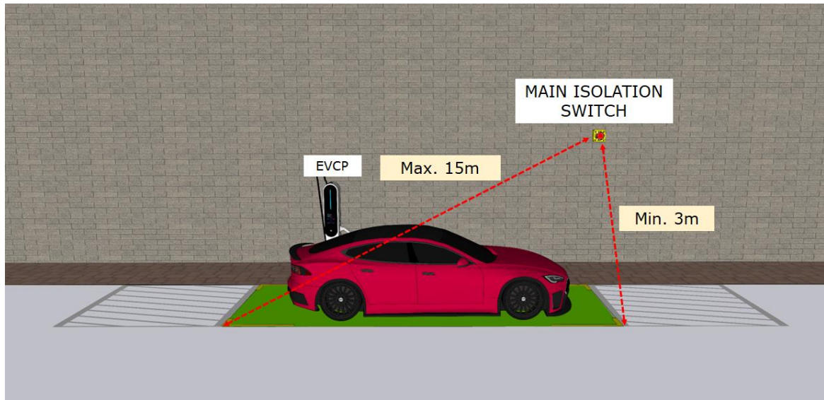
Rajah 10: Kedudukan Suis Pengasingan Elektrik Utama
